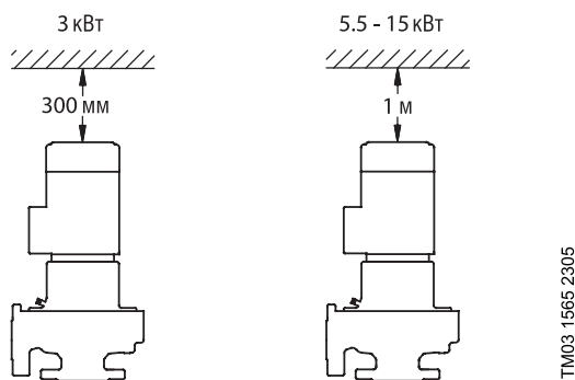
Рис. 9 Вертикальная установка
